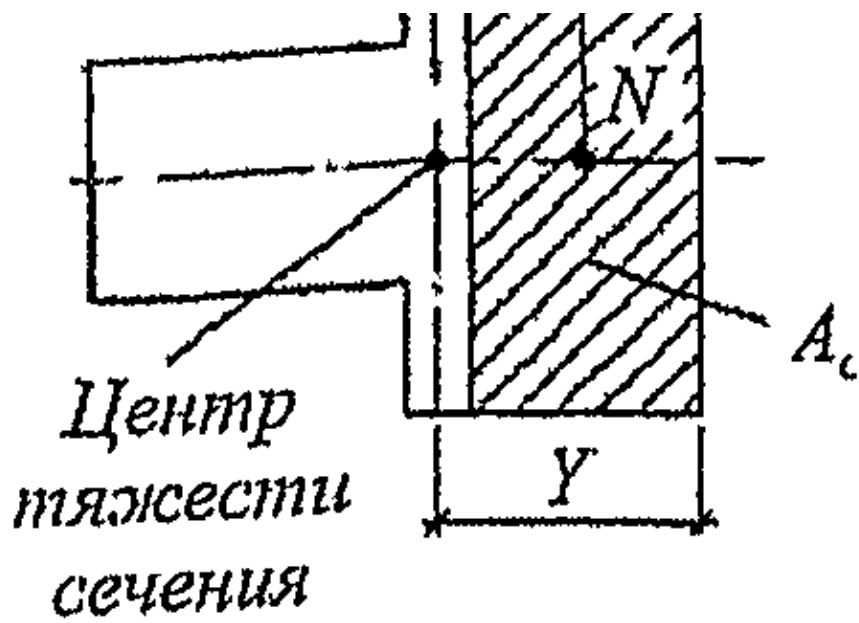
Рисунок 5 – Внецентренное сжатие
