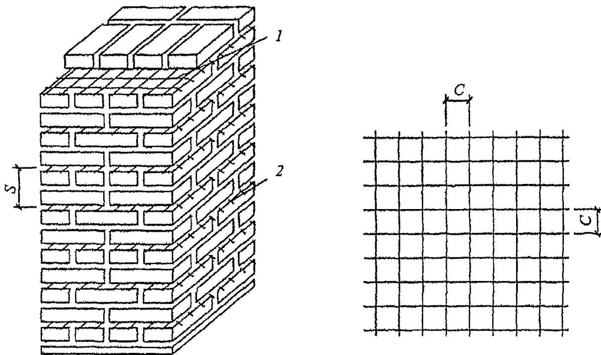
Рисунок 11 – Поперечное (сетчатое) армирование каменных конструкций
