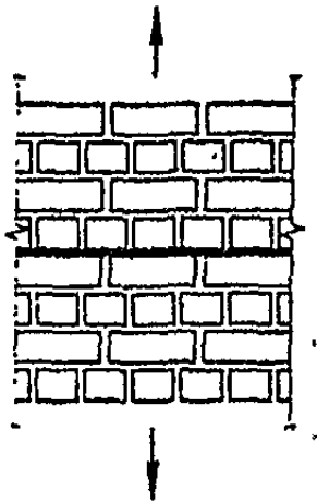
Рисунок 1 – Растяжение кладки по неперевязанному сечению
