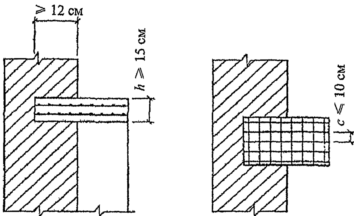
Рисунок 13 – Железобетонные распределительные плиты
