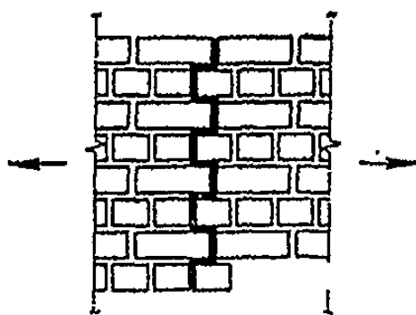
Рисунок 2 – Растяжение кладки по перевязанному сечению
