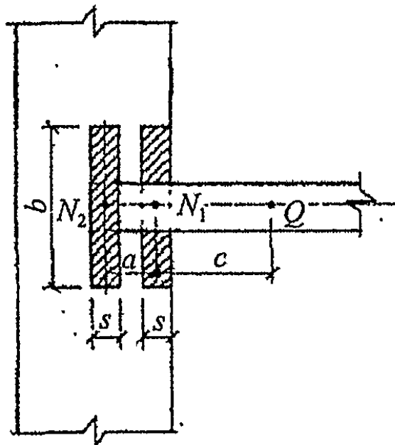
Рисунок 14 – Расчетные схемы заделки консольных балок
