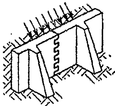
Рисунок 3 – Растяжение кладки при изгибе по перевязанному сечению
