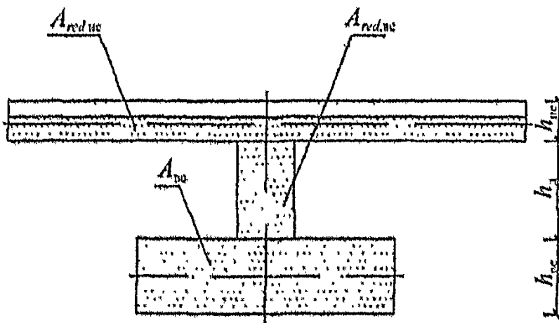
Рисунок 10 – Приведенное сечение рассчитываемого фрагмента стены
